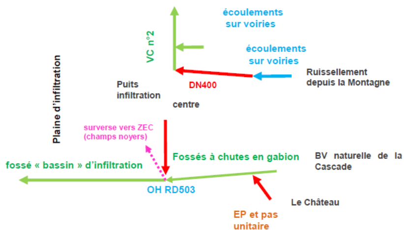
Synoptique du fonctionnement des écoulements pluviaux.
